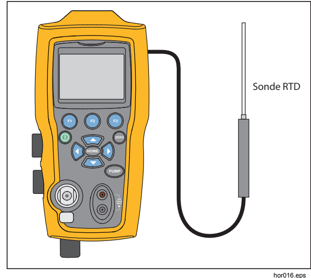
Figure 7. Mesure de température avec une sonde RTD
