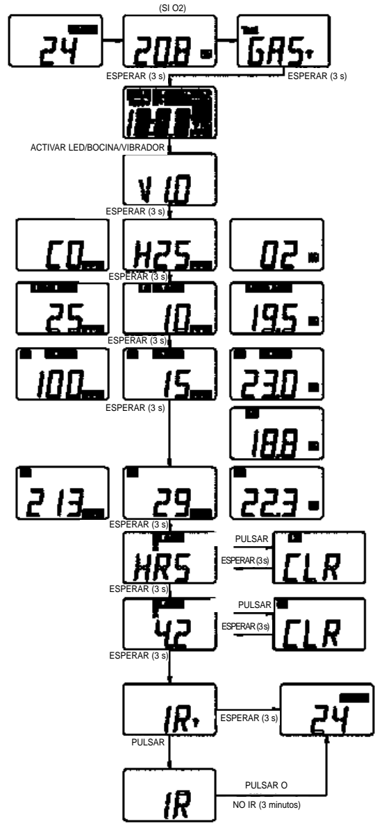
Figura 2-5. Acceso al diagrama de flujo de las páginas del Altair
