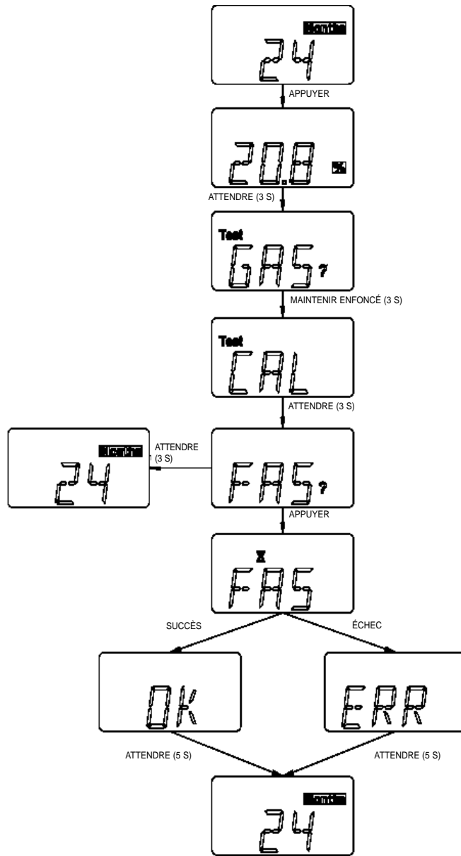
Figure 4-2 Diagramme de calibrage (oxygène)
