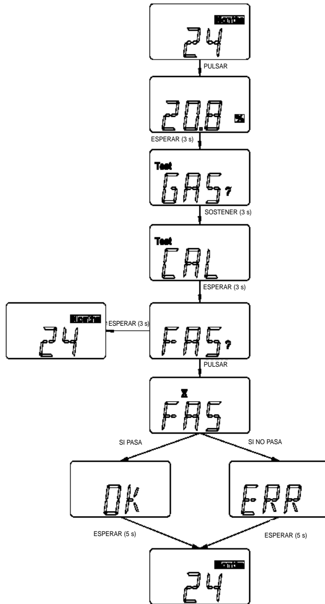
Figura 4-2 Diagrama de flujo de calibración (oxígeno)
